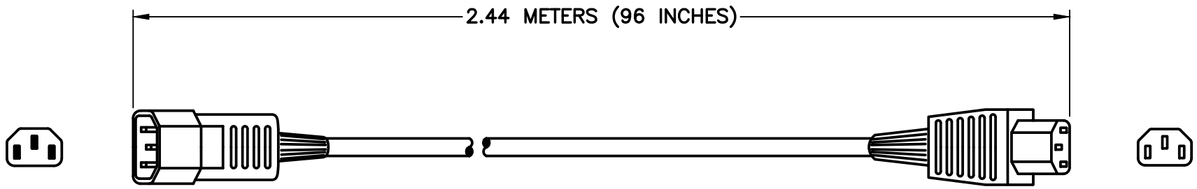
IEC 60320 C-14
